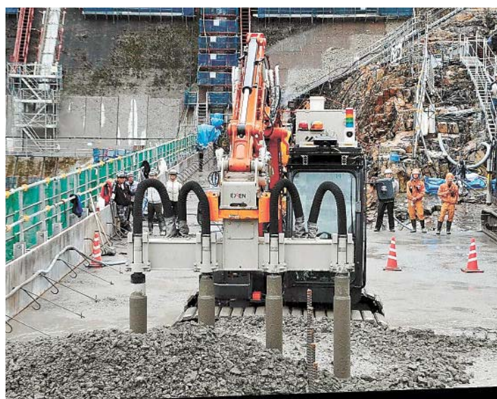
自動運転でコンクリの締め固めを行う重機＝可児郡御嵩町、新丸山ダム工事現場
